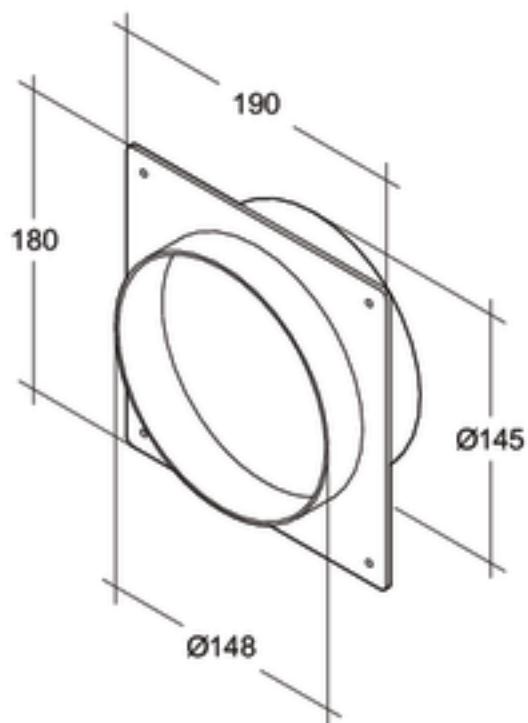
Maueranschlußstutzen rund 150 mit Klappe Material: Kunststoff
